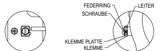
DETAILLIERTE FRONTANSICHT
